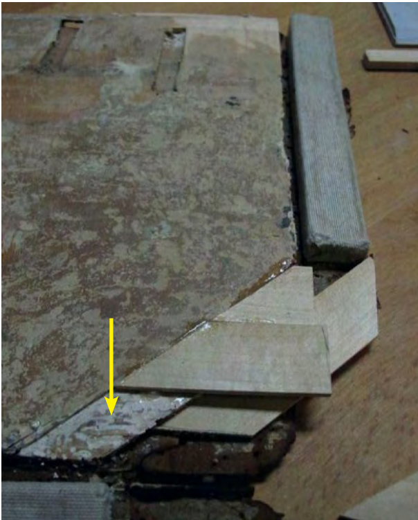
en cours: retrait de matière dans le bois original afin d'obtenir une meilleure surface de collage (flèche jaune). Des pièces très fines de bois neuf sont intégrées sur et sous l'original, en contrariant l'orientation de leurs fibres, afin d'améliorer la stabilité du comblement.
