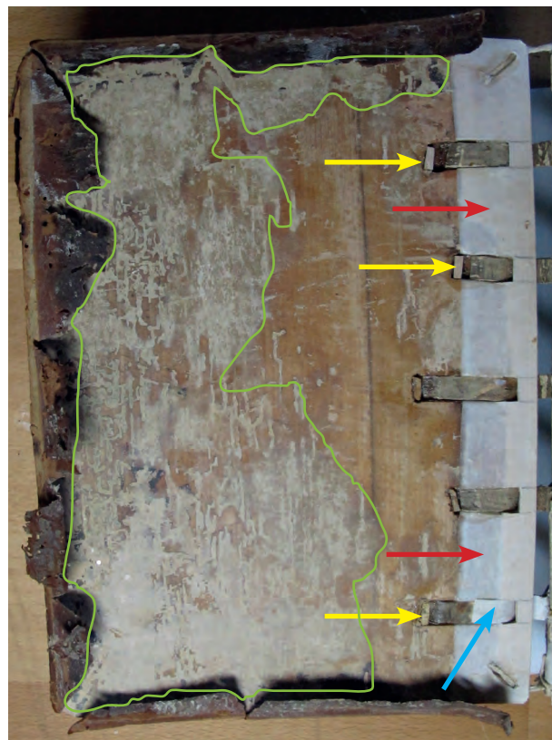
en cours: Meilleure stabilité après comblement des zones vermoûlues (en vert) ; bande rempliée de parchemin permettant une consolidation supplémentaire du mors (flèche rouge) ; nouvelles chevilles (flèches jaunes); renfort du nerf rompu (flèche bleue)
