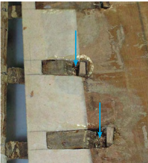
en cours: Afin d'éviter des dommages ultérieurs de l'ais, le plat a été légèrement décalé en direction de la gouttière. Cette opération a entraîné un décalage des lanières dans les passages de l'ais; les nerfs ont donc été collés et ne sont plus maintenus par les chevilles. Les chevilles sont toutefois remises dans leur position d'origine.
